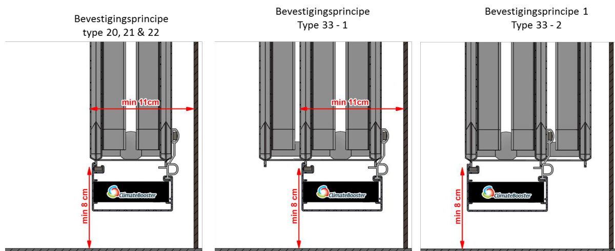
Figuur 1 - Benodigde vrije ruimte Radiator Pro
